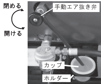
図3-5 手動エア抜き弁使用方法
