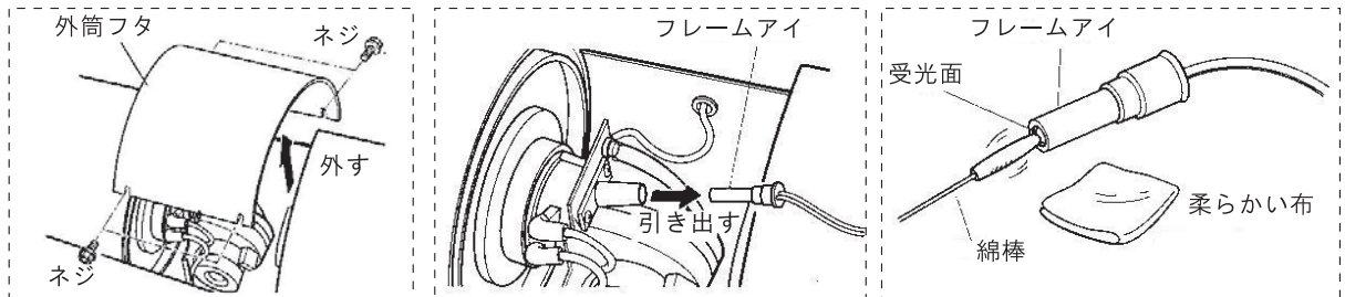
図5-1-2 フレームアイの点検方法
