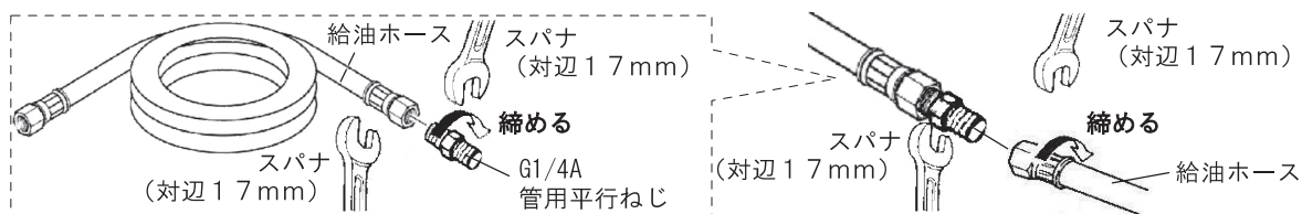
図3-4-4 給油ホースの延長方法
