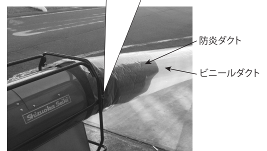
図3-2-1 ダクトの取付け方法
