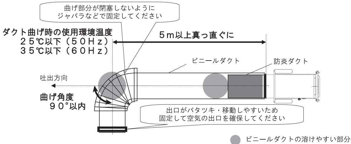
図3-2-2 ビニールダクト使用時の設置例（上から見た図）
