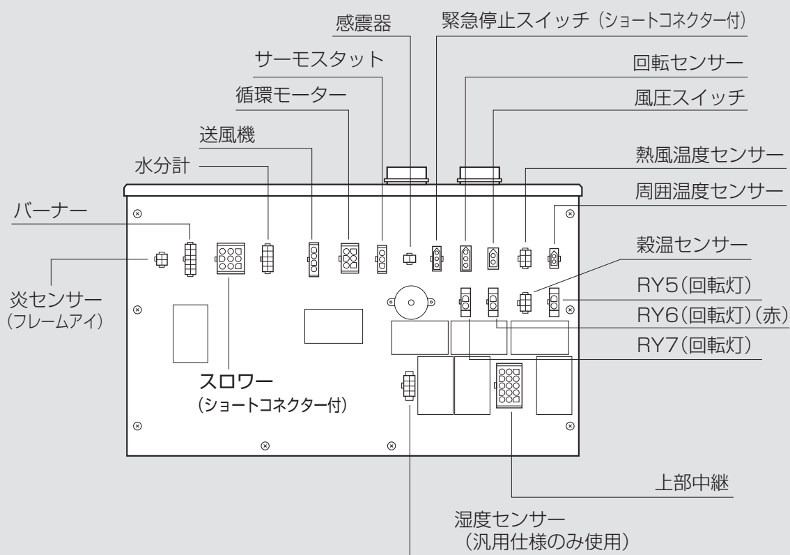
コントロールボックス下面から見たところ
