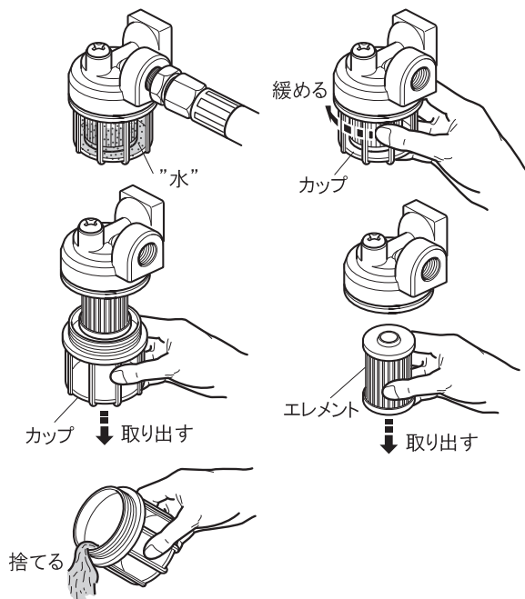
図5-1-A エレメントの点検方法
