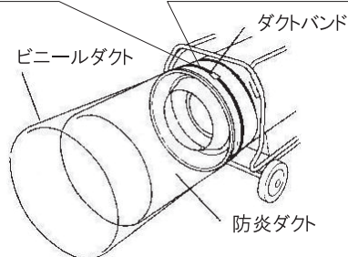
図9-2-A ダクトの取付け方法
